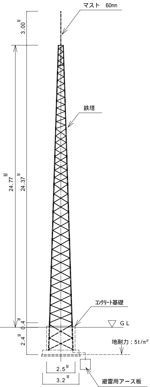
立面図 S=1/200
